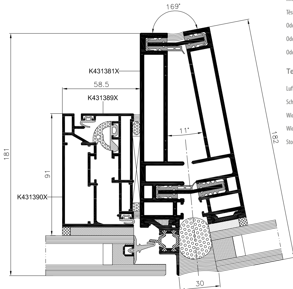
Průřez sloupku s výkyvným oknem
