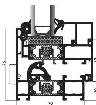
okno otvíravé – řez
